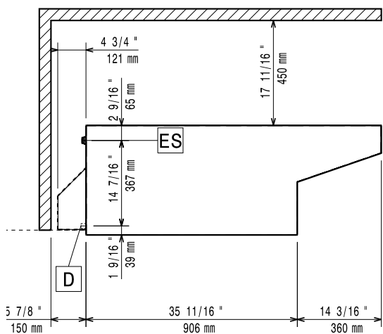
Felülnézet
