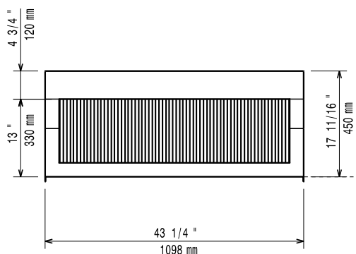
Oldalnézet
